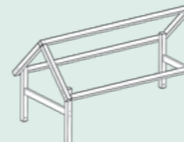
Dachaufbau für Einzelbett und halbhohes Bett B/H/T 222/119/116 cm
