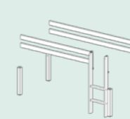
Erweiterungs-Set für halbhohes Bett, Basisbett vorausgesetzt, best. aus: Verlängerungspfosten, Absturzicherung und gerader Leiter
